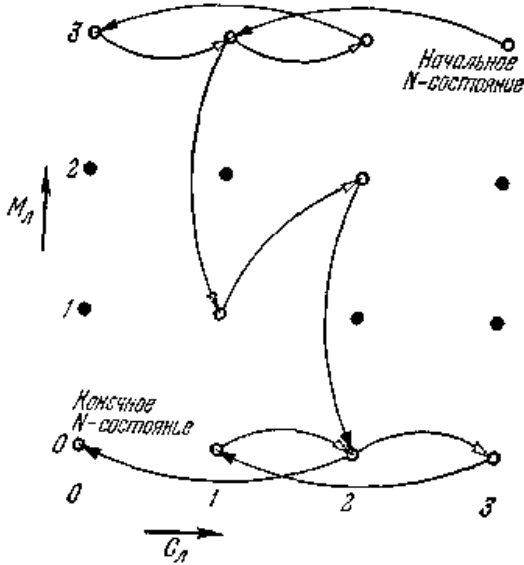
Рис. 10.2. Пространство N -состояний для элементарной задачи о миссионерах и людоедах.
