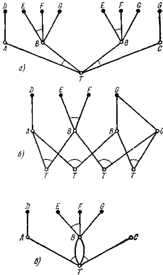
Рис. 10.10. Представление задачи T в виде пропозиционального дерева (а), графа доказательства определений (б) и графа вывода (в).
