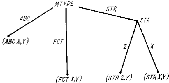
Рис.10.12. Пример дискриминационной сети.
