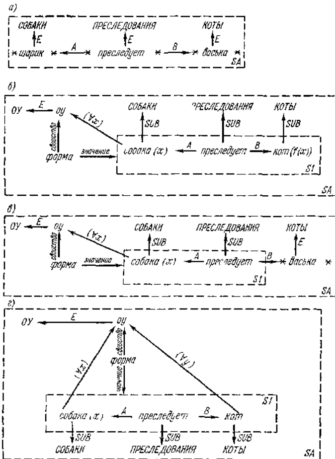
Рис. 10.24. К разбиению семантической сети на пространство.
