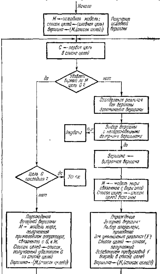
Рис. 1. Схема работы планирующей системы P3.
