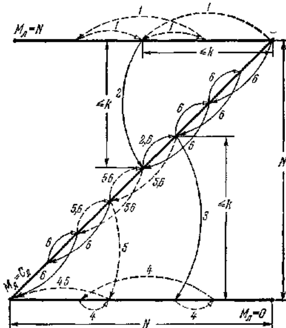
Рис. 3. Схемы решений обобщенной задачи о миссионерах и людоедах в Z области. Цифры у дуг соответствуют пунктам в тексте.
