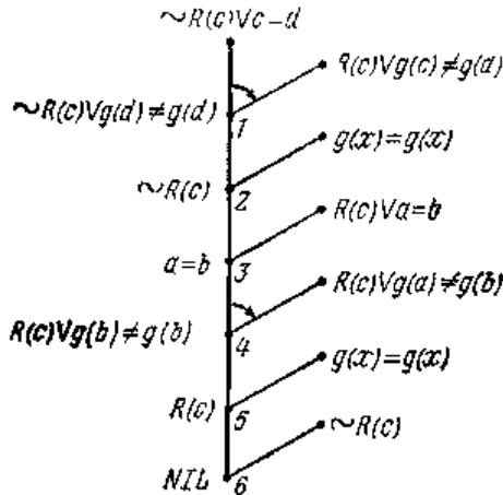
Рис. 7. Линейное опровержение с резольвцией и парамодуляцией.
