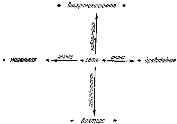
Рис.11. Представление атрибутивных отношений.
