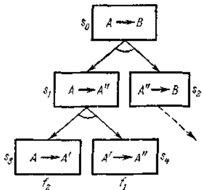
Рис. 8. Пропозициональный граф, соответствующий процессу редукции.
