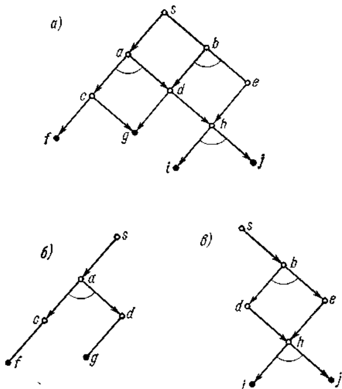
Рис. 4. Аддитивный пропозициональный граф ( а ) и его решающие графы ( б , в ).
