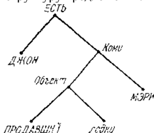
Рис. 8. Представление структуры предложения в виде бинарного дерева.
