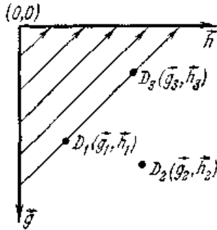
Рис. 2. Геометрическая интерпретация диагональной поисковой стратегии
