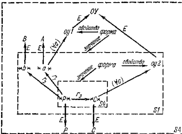
Рис.16. Представление последовательности логических кванторов, (\forall a \in A)(\exists b \in B)(\forall c \in C)(p(a,b,c)) .
